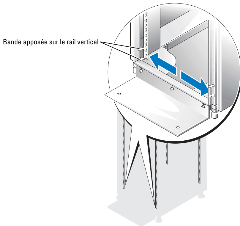
Figure 1-4. Marquage des rails verticaux
