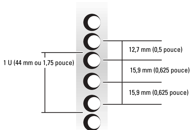
Figure 1-11. Espacement des trous sur un rack universel à 2 montants et châssis ouvert
